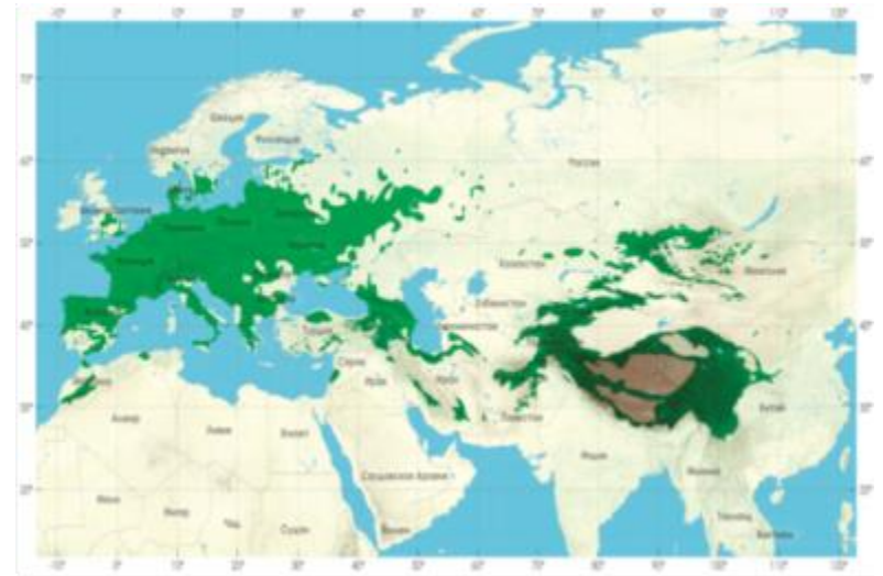
Рис. 2. Гнездовой ареал горихвостки-чернушки ( Phoenicurus ochruros ). В.А. Федоренко (2018)
