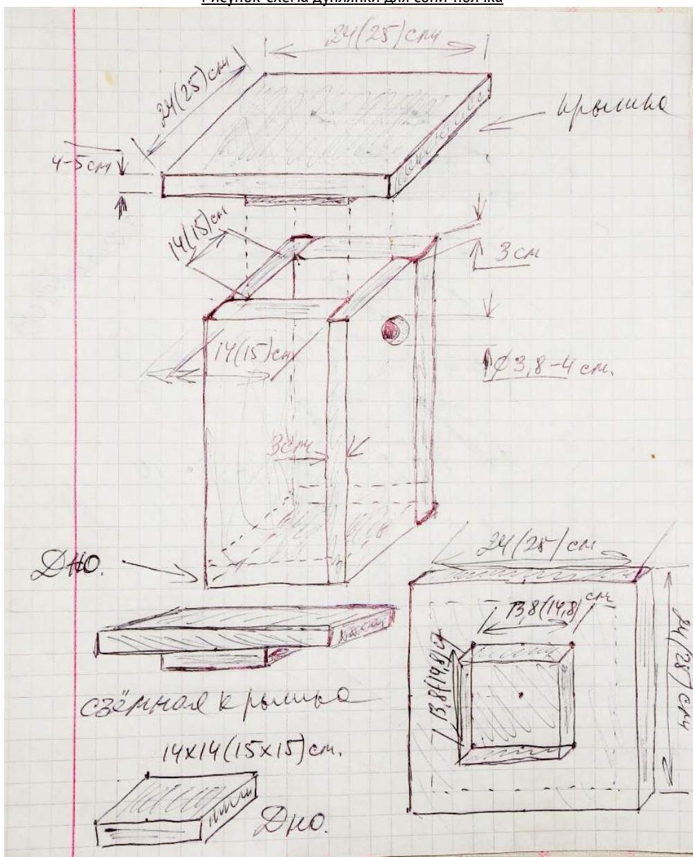
Рисунок-схема дуплянки для сони-полчка
