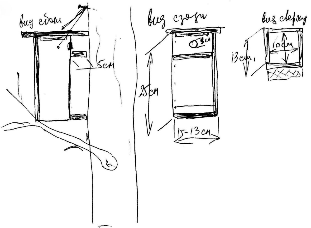
Рисунок-схема дуплянки для лесной сони
